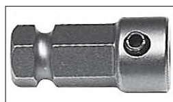
Bussola portamaschio con grano di bloccaggio (esagono 12 mm). Tap holder with locking dowel (hex 12 mm).
