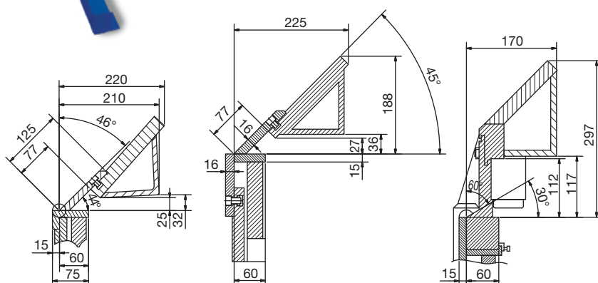
Dimensioni E-Serie
