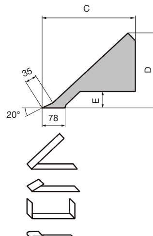
Dimensioni ganascia di piegatura MSBM
