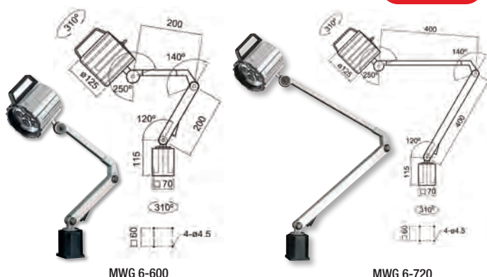
MWG 6-600
