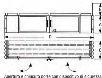
Apertura e chiusura porte con dispositivo di sicurezza
