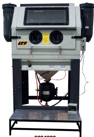
3204990 Sabbatrice KUS con serbatoio a pressione
